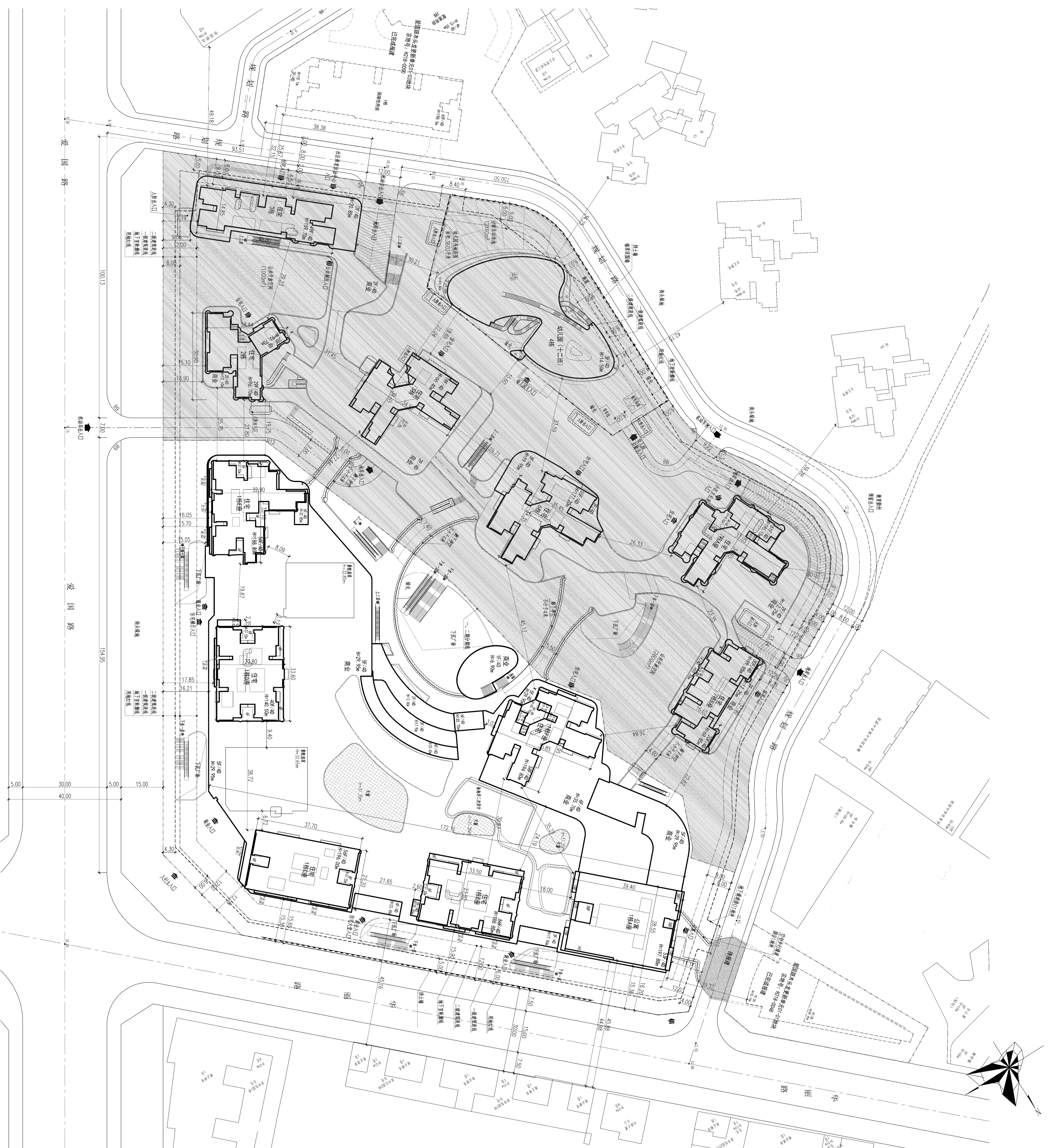
二期总平面图 (公告版) 1:500
